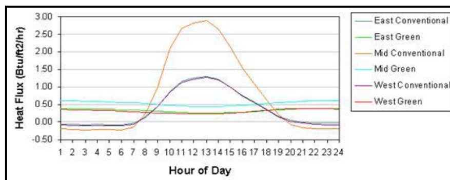
شکل ۱- متوسط گرمایش روزانه یک ساختمان (۴ جولای تا ۱ سپتامبر ۲۰۰۵)
