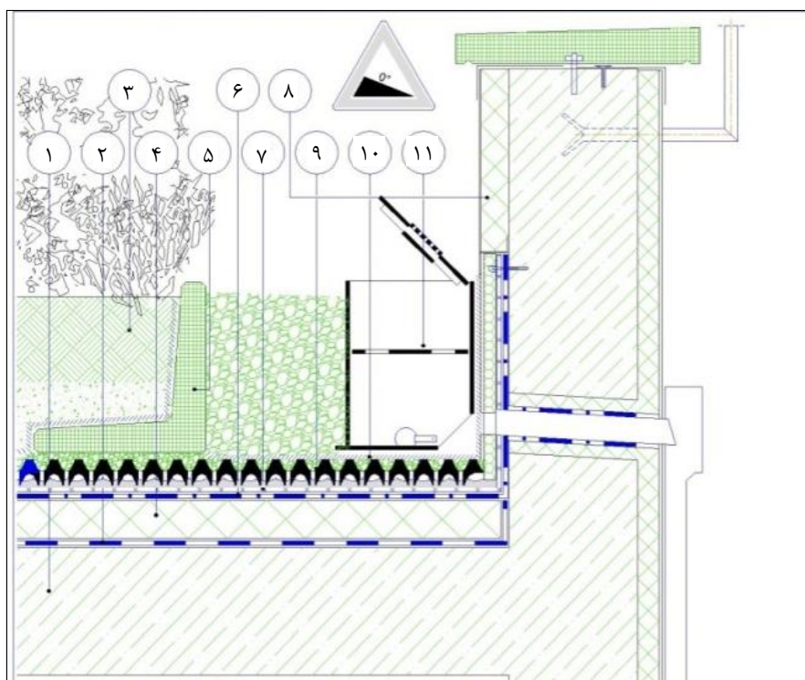
شکل ۵-۲- مقطع بام سبز نیمه فشرده، مأخذ: شرکت دیادم
