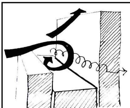
شکل ۳-۴ - حلقه جریان هوای ایجاد شده میان دو ساختمان
