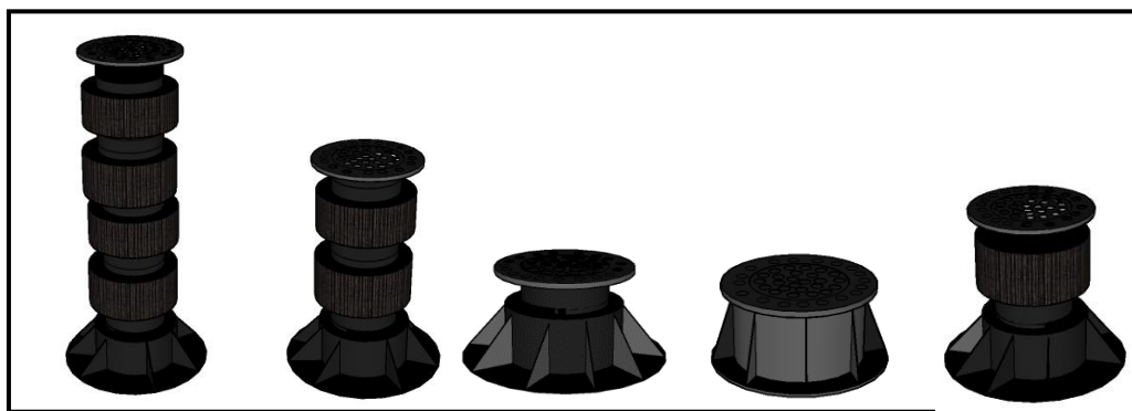
شکل ۲-۱۰- نمونه‌هایی از پایه برای نصب کفپوش و روش نصب آن
