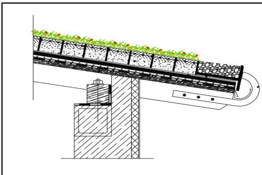
شکل ۲-۱۲- اجرای بام سبز گسترده شیب‌دار
