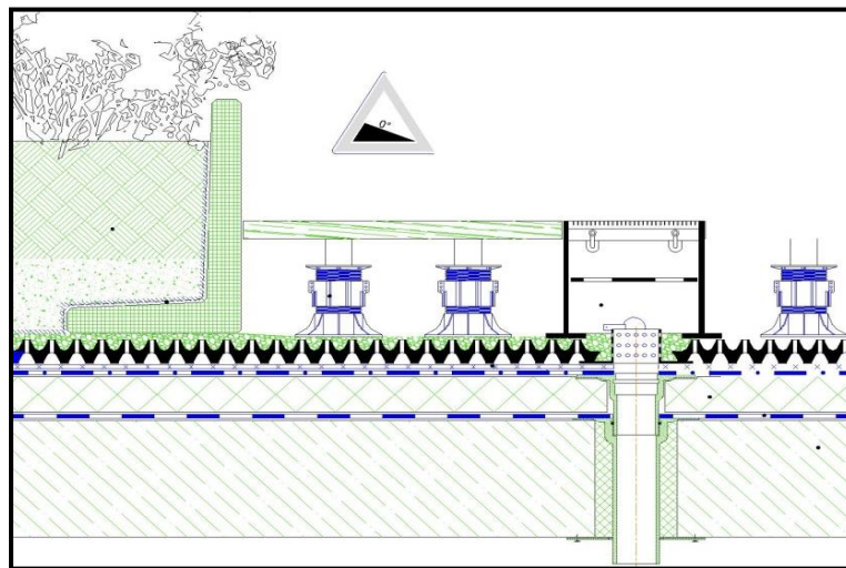
شکل ۲-۹- جزئیات نصب کفپوش در بام سبز
