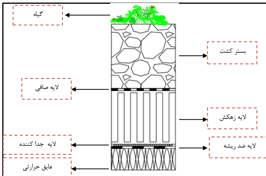
شکل ۱-۸- اجزای بام سبز و مراحل اجرای آن
