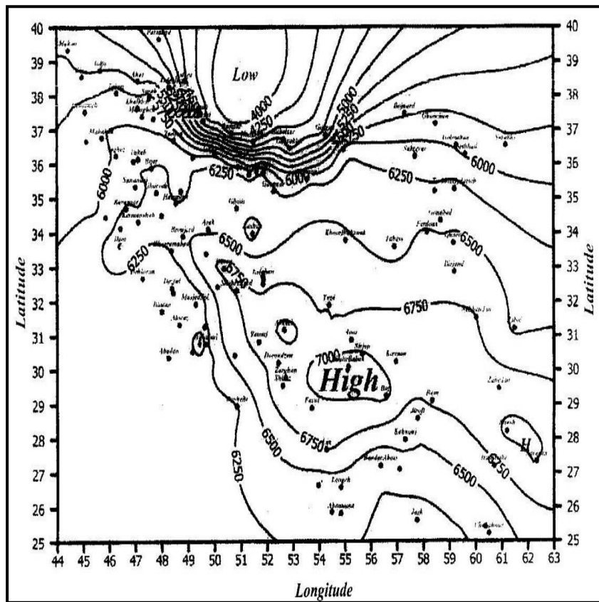
پ.۲-۳- انرژی خورشیدی دریافتی بر روی سطوح افقی در طول یک سال در ایران (MJ/m 2 ), صفايي ۲۰۰۵
