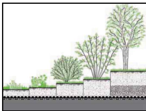
شکل ۱-۱- ضخامت لایه خاک و نوع گیاهان انواع بام سبز
